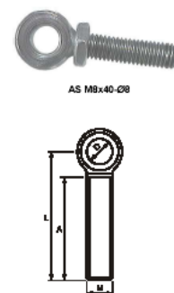
Rys. 27. Śruba oczkowa.
