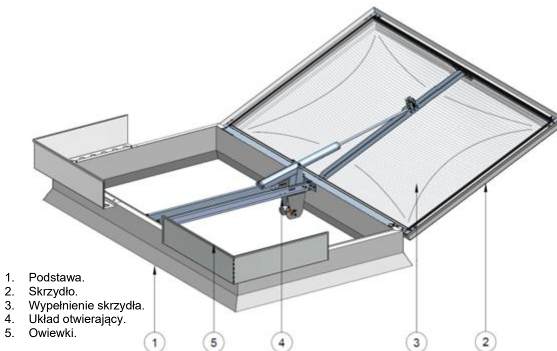
Rys. 1. Budowa klapy oddymiającej mcr ULTRA THERM. (Przykład z układem otwierającym JOFO).
