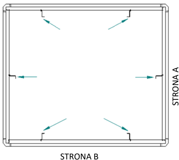
Rys. 35. Montaż uchwytów kierownicy.
