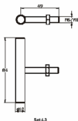
Rys. 25. Śruba „T”.
