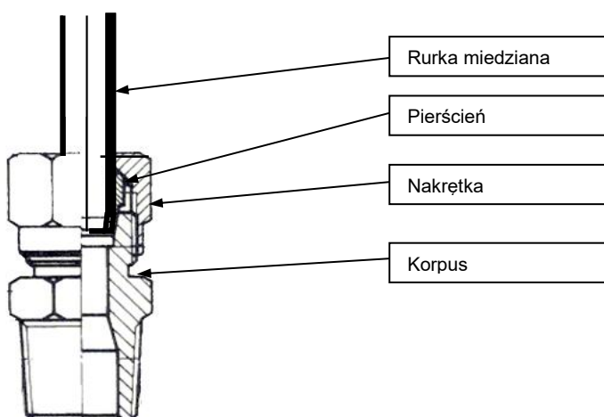
Rys. 47. Połączenie śrubunku z rurką miedzianą/stalową.
