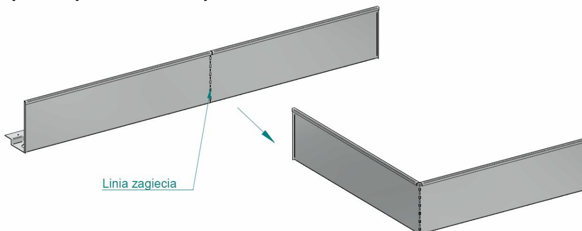
Rys. 33. Zagięcie owiewek.
